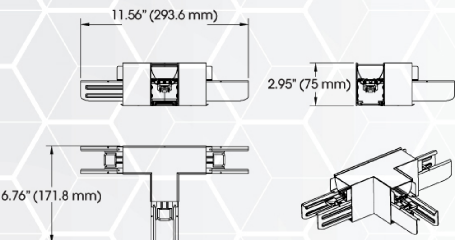
T-CONN
