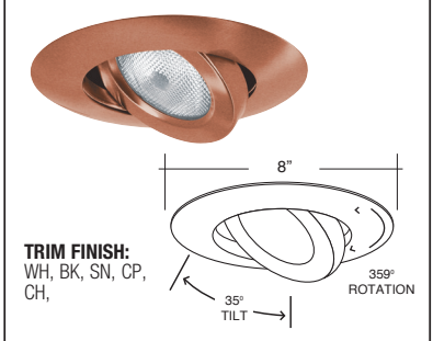
B1663CP PAR36 GIMBAL RING
